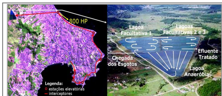
Fonte: CASAN, 2004, modificado pela autora Figura 5 – Funcionamento da ETE Potecas
