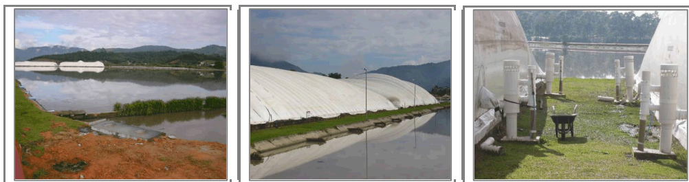
Figura 6 – Tanques cobertos com lona de PVC
