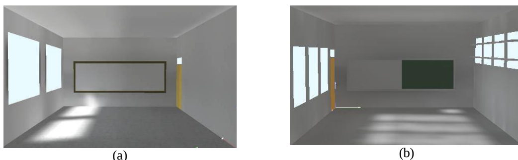
Figura 5 - Simulação da luz natural na sala 06 (a), considerando as condições reais existentes para o dia 21 de dezembro às 9h. Simulação da luz natural na sala 09 (b), considerando as condições reais existentes no dia 21 de junho às 15h.
