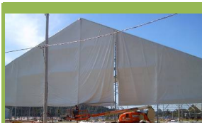
Figura 3 - Estrutura desmontável permite o reaproveitamento dos materiais
