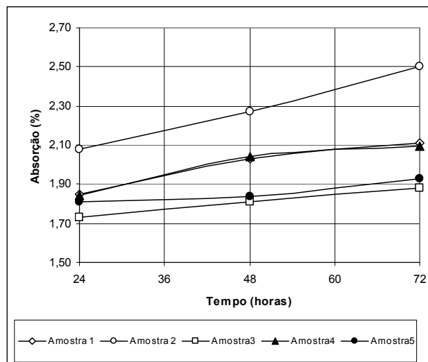
Gráfico 2 – Absorção por imersão
