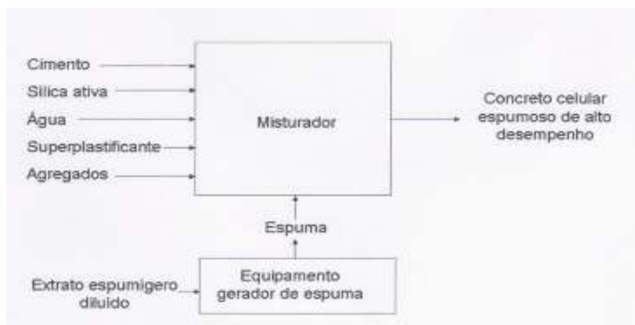
Figura 1 – Diagrama esquemático da produção do concreto celular espumoso de alto desempenho
