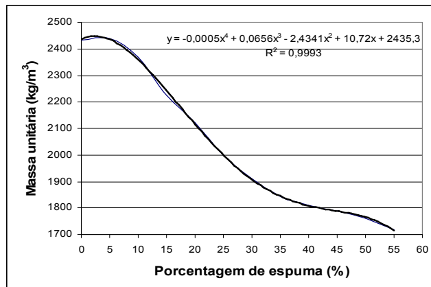
Gráfico 1 – Curva para determinação da dosagem de espuma
