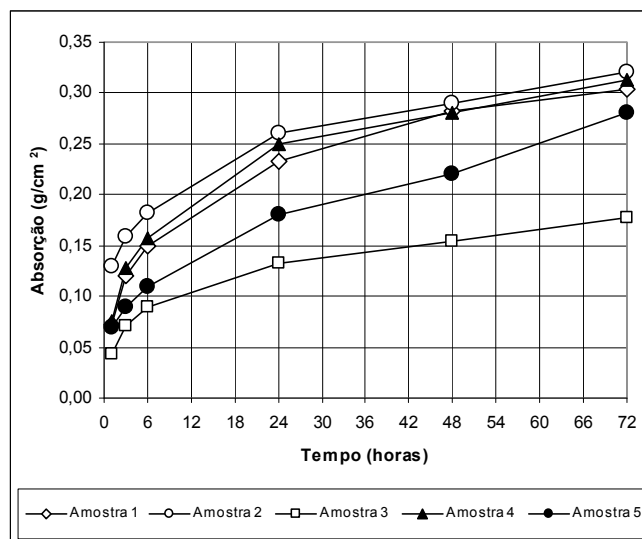
Gráfico 3 – Absorção por capilaridade
