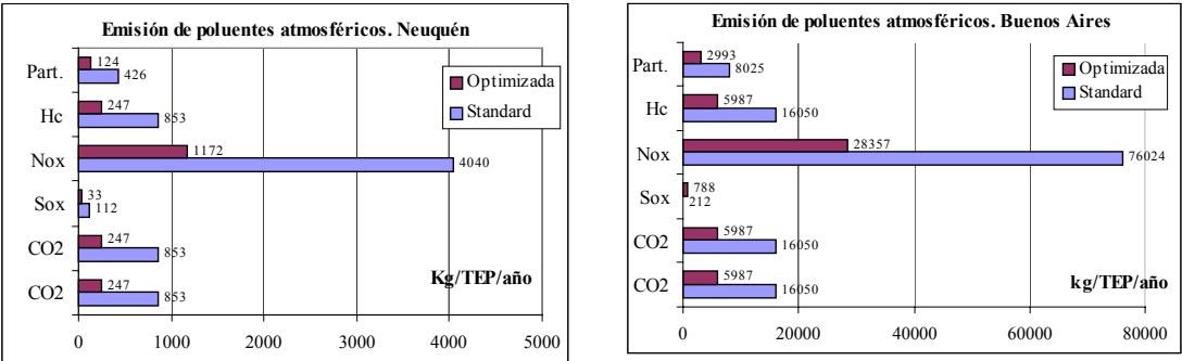
Figura 4. Emisión de poluentes atmosféricos. Neuquén y Buenos Aires. Original y Optimizada.
