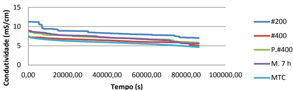
Figura 4 – Condutividade elétrica versus tempo de CH/CB400
