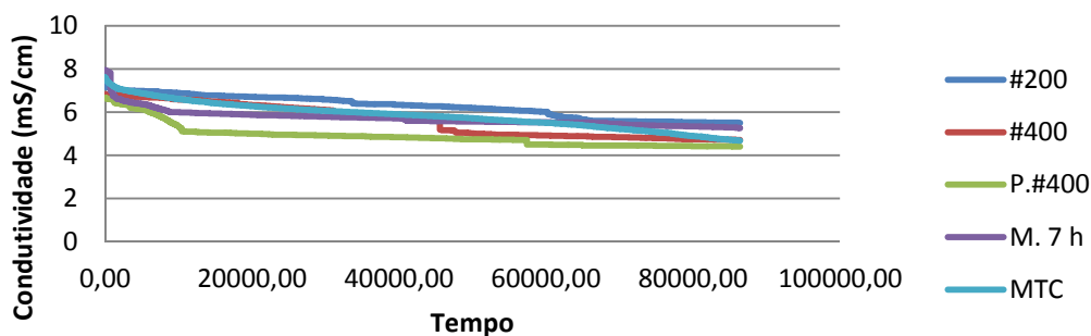
Figura 3 – Condutividade elétrica versus tempo de CH/CB300
