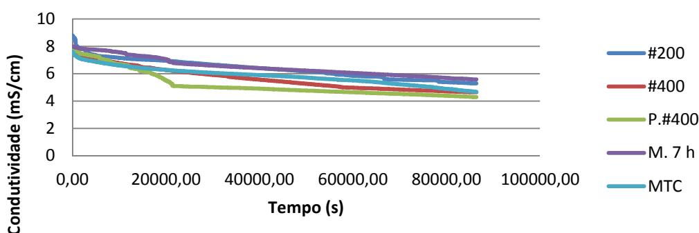
Figura 6 – Condutividade elétrica versus tempo de CH/CB600
