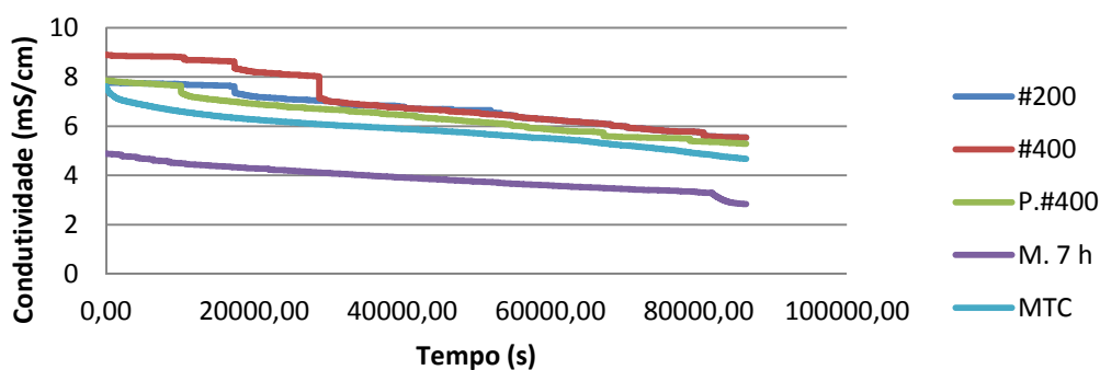
Figura 2 – Condutividade elétrica versus tempo de CH/CAN
