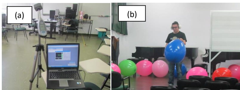
Figura 1. Montagem dos equipamentos de medição acústica (a); geração do impulso - estouro de balão (b)
