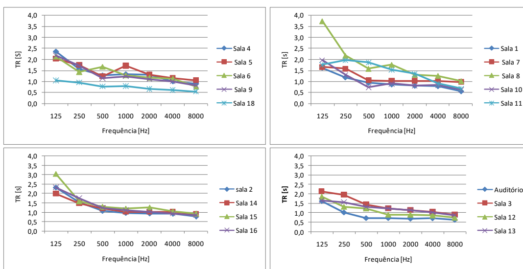
Figura 2. Valores de tempo de reverberação (TR) nas bandas de frequência de oitava (125-8.000 Hz) para cada grupo de recintos
