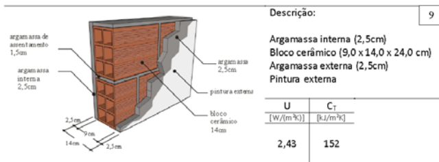
Figura 10: Parede empregada na habitação
