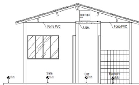
Figura 3: Corte transversal
