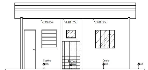
Figuras 2: Corte longitudinal
