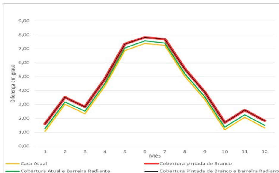
Figura 13 - Diferença entre as temperaturas máximas das casas atual e com as intervenções no dia típico de verão em Cuiabá-MT
