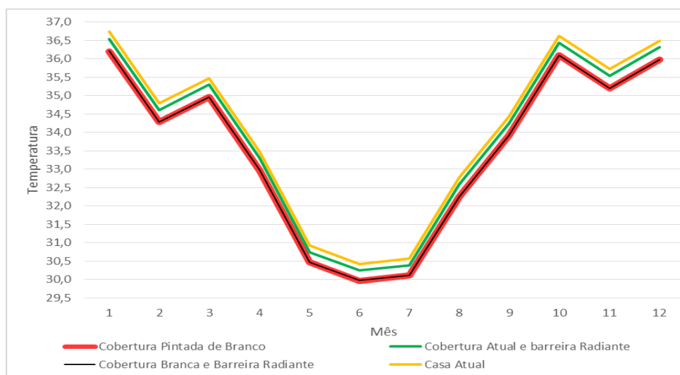
Figura 12 – Temperaturas internas máximas da casa atual e com as intervenções (pintura da cobertura na cor branca, cobertura atual+colocação de barreira radiante e pintura da cobertura na cor branca+colocação de barreira radiante).
