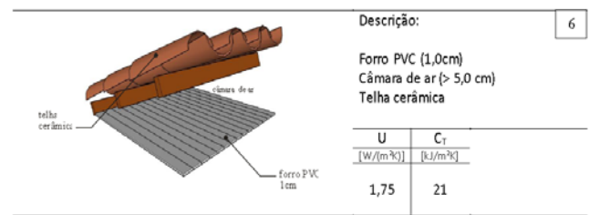
Figura 11: Cobertura empregada na habitação
