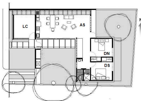
Figura 1 – Planta de La vivienda VBP-1
