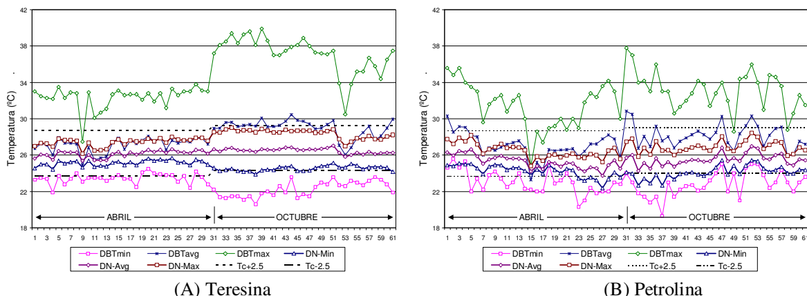
Figura 6: Temperatura max, med y min en DN y ambiente exterior en abril y octubre con limites de confort de referencia.
