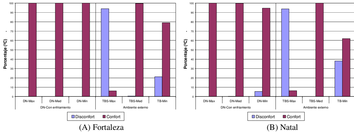
Figura 9: Porcentajes de confort/discomfort en el SPEEI (DN-con enfriamiento) y ambiente exterior.
