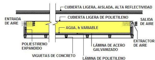
Figura 2– Esquema del SPEEI
