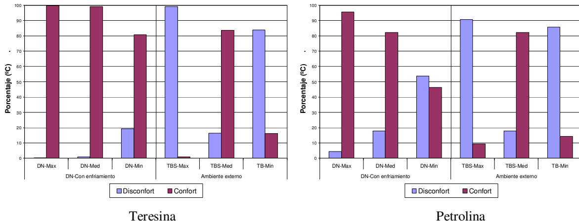
Figura 8: Porcentajes de confort/discomfort en el SPEEI (DN-con enfriamiento) y ambiente exterior.
