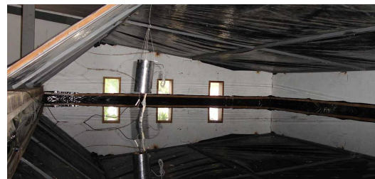
Figura 3– El techo-estanco sobre dormitorios
