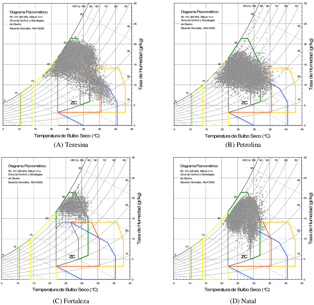
Figura 5: Datos de temperatura y humedad horarios sobre diagrama psicrométrico y estrategias de diseño bioclimático.
