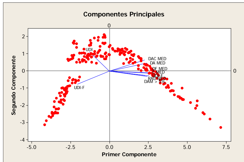
Figura 9 – Componentes principales: gráfico de dos dimensiones.
