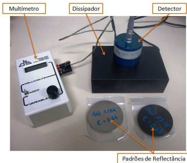
Figura 6. Componentes do emissômetro.
