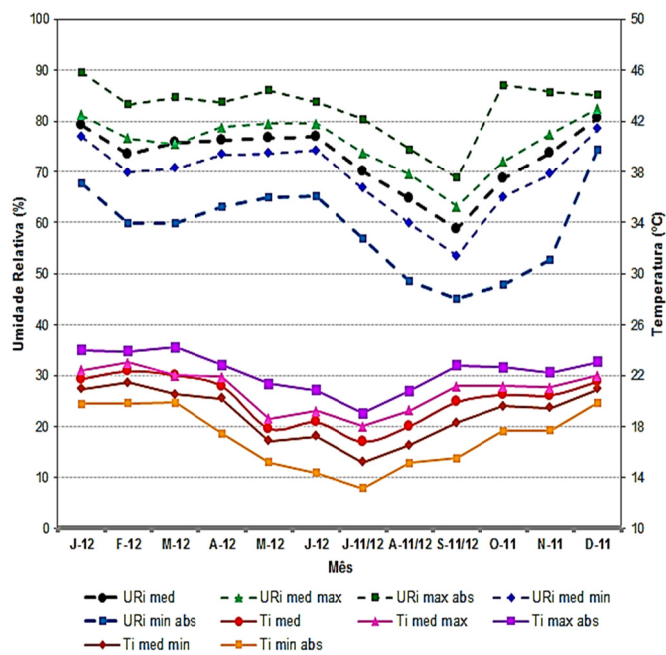
Figura 4 – Capela da Ceia – Climograma interno. Período 18/07/2011 a 21/10/2012.
