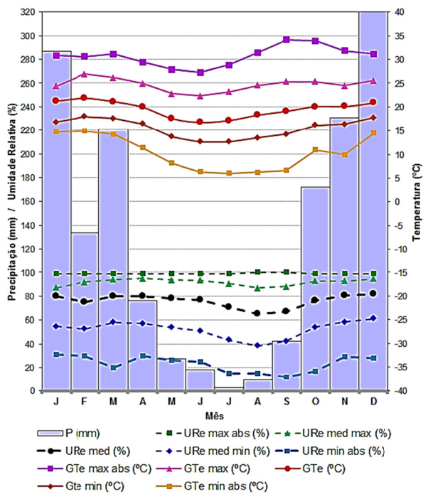
Figura 3 – Ouro Branco – Climograma período 2006-2012.
