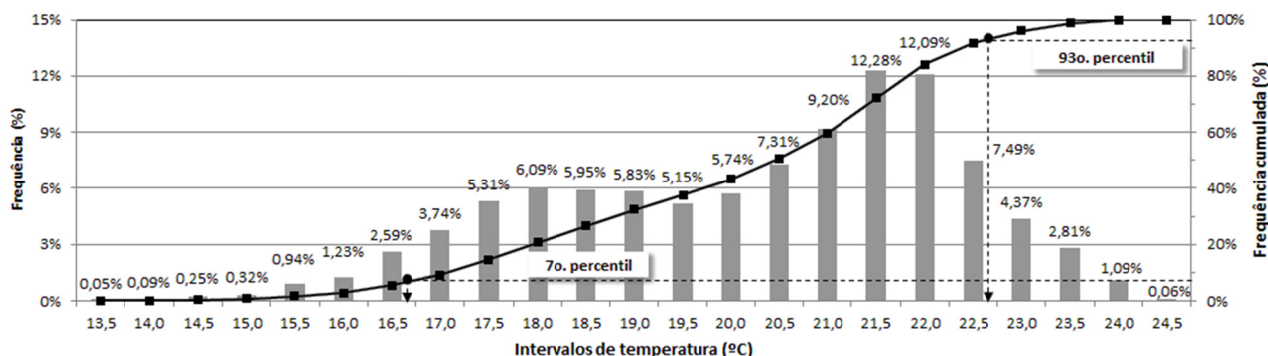
Figura 5 – Capela da Ceia – histograma de frequências de temperaturas.
