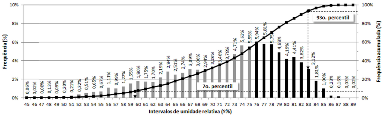
Figura 6 – Capela da Ceia – histograma de frequências de umidade relativa.
