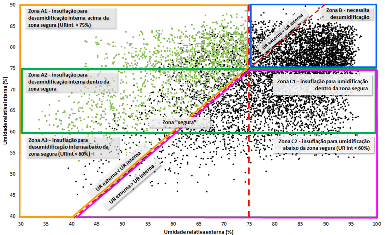
Figura 7 – Capela da Ceia – umidade relativa externa (médias horárias 2006-2012) versus umidade relativa interna (médias horárias 2011-2012). Ocorrências c/ T_e < 25^\circ\text{C} , correspondendo a 94,5% das ocorrências. Em verde, pontos com W_e < W_i .
