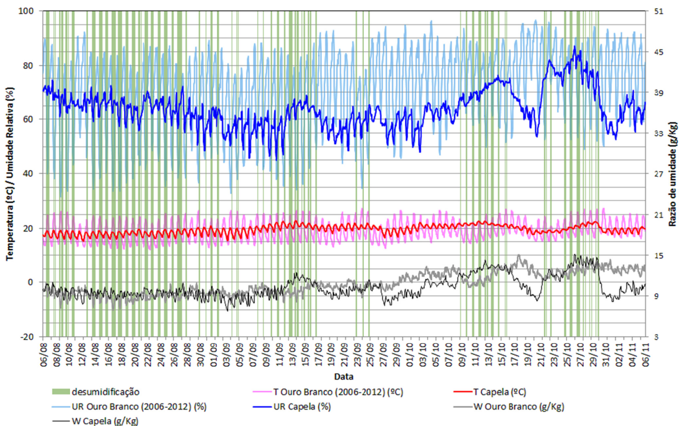
Figura 8 – Capela da Ceia – horários com desumidificação aplicável. Período: 06/08/12 a 05/11/12 (primavera). Dados internos, médias horárias, período 2011-2012 versus dados externos, médias históricas, período 2006-2012.
