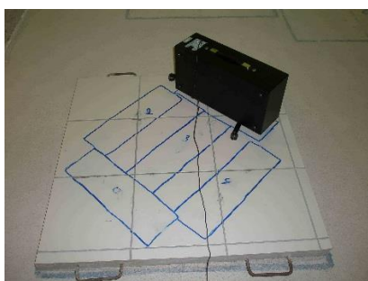
Figura 4 – Posição da máquina de impacto sobre contrapiso, câmara superior.
