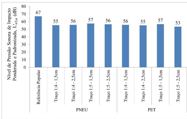
Figura 6 – Dados do L'_{nT,w} para contrapiso em cerâmica popular.
