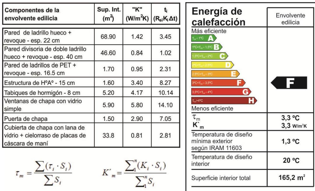
Figura 8: nivel de eficiencia energética de la vivienda para calefaccionar s/Norma IRAM 11900
