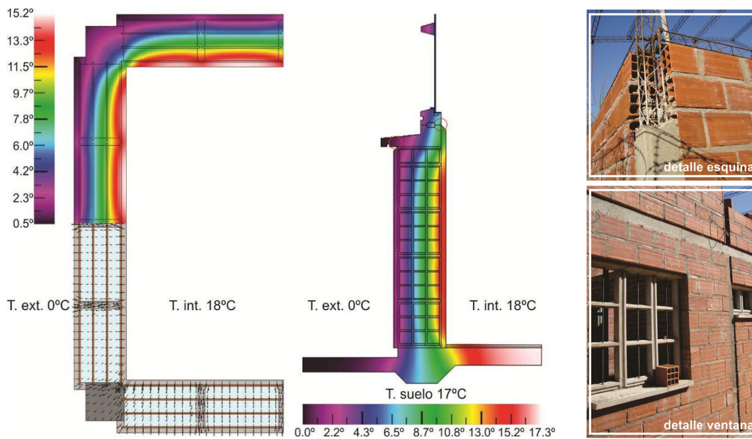
Figura 6: simulación de puente térmico para dos soluciones constructivas, encuentro en esquina entre pared y columna (izquierda) y encuentro entre pared con carpintería de H^{\circ}A y platea de H^{\circ}A (derecha).
