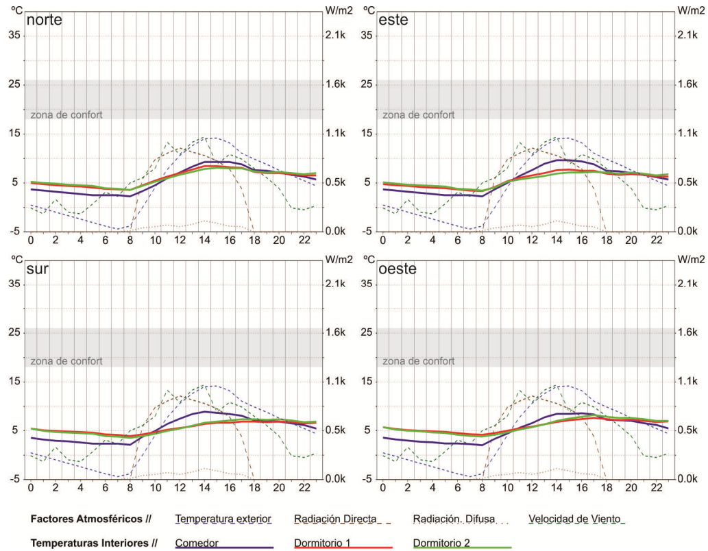
Figura 4: temperatura horaria promedio de los locales para un día de invierno, según distintas orientaciones.
