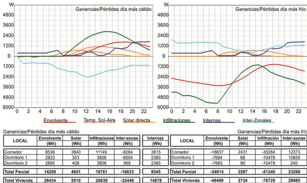
Figura 5 y Tabla 3: promedio de las ganancias y pérdidas horarias expresadas en Watts, de los locales seleccionados, para los días extremos de verano e invierno.
