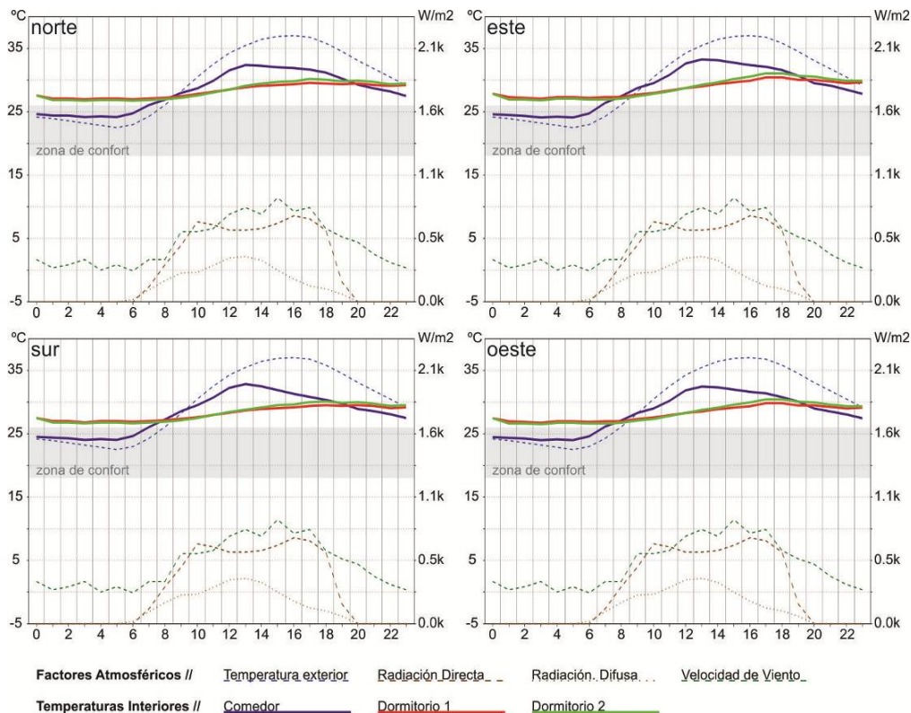
Figura 3: temperatura horaria promedio de los locales para un día de verano, según distintas orientaciones.
