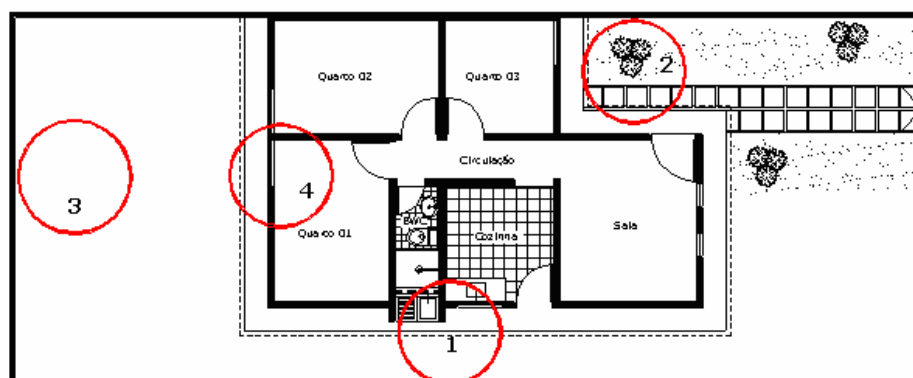
Figura 5 – Planta baixa original e expansões previstas pelos construtores.
