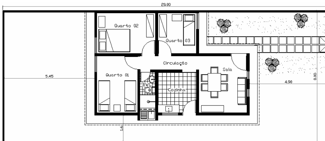
Figura 2 - Planta baixa (com mobília proposta) de unidade original do Conjunto Osman Loureiro.
