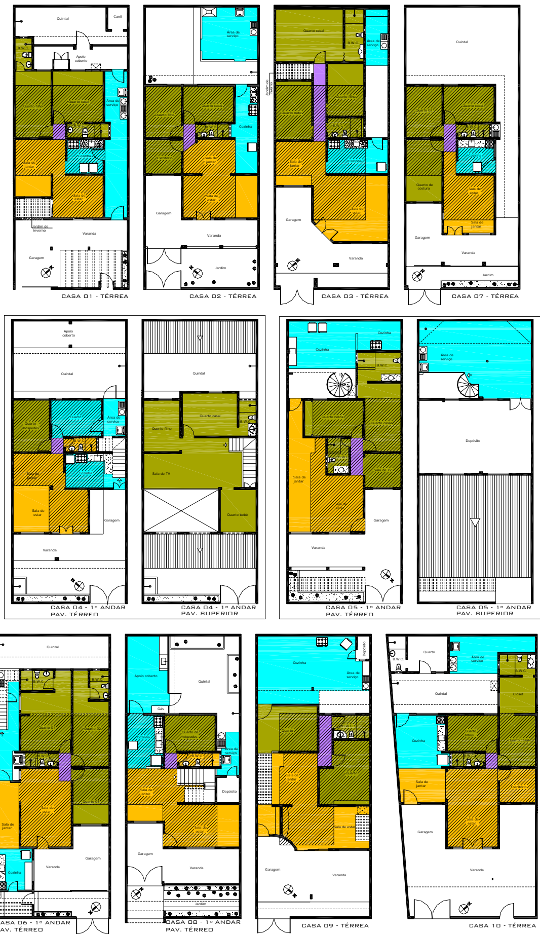
Figura 4 – Reformas das 10 unidades analisadas (a parte hachurada representa a projeção da casa original; azul – serviço; ocre – social; verde – íntimo; roxo - circulação).
