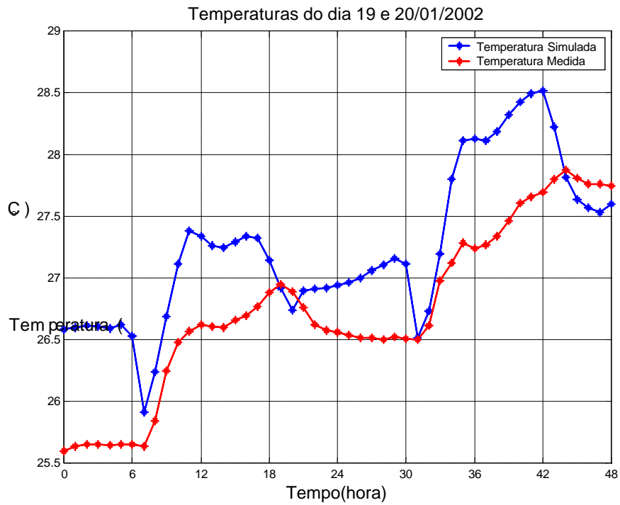
Figura 4 - Gráfico da temperatura da sala-teste.
