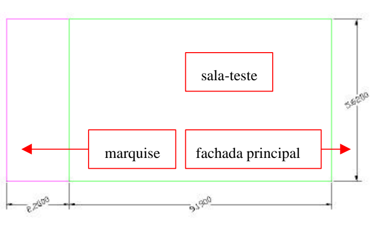
Figura 1 - Croqui da sala-teste gerado através do arquivo .dxf.
