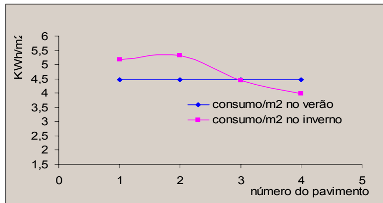
Figura 4 - Gráfico do Consumo/m 2 para orientação 100^\circ , alterando o pavimento
