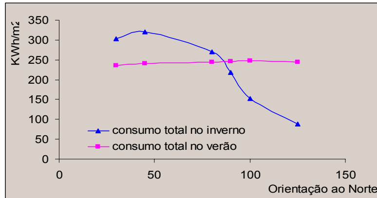
Figura 1 – Gráfico do Consumo Total com variáveis médias em função da orientação
