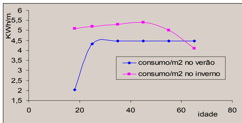
Figura 6 – Gráfico do Consumo /m 2 para orientação 100°, alterando a idade
