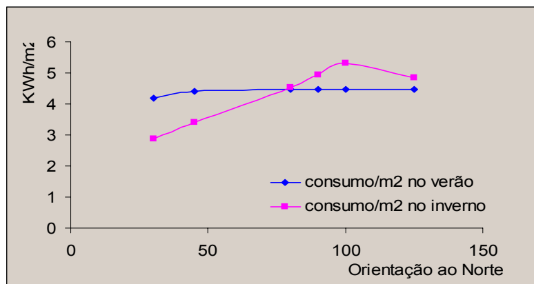
Figura 2 – Gráfico do Consumo /m 2 com variáveis médias em função da orientação
