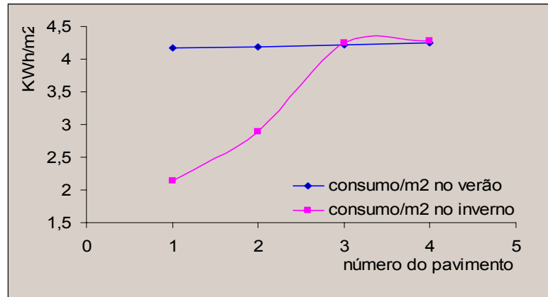
Figura 3 – Gráfico do Consumo /m 2 para orientação 30^\circ , alterando o pavimento
