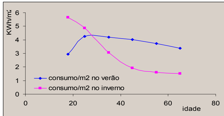
Figura 5 – Gráfico do Consumo /m 2 para orientação 30°, alterando a idade
