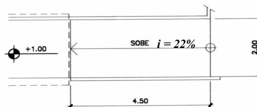
Fig. 4 – Planta rampa 1 – Escola C Fonte: Autor, 1998
