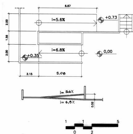
Fig.1 – Planta rampa de Entrada Escola A
