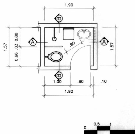
Fig. 6 – Planta do sanitário adaptado de forma incorreta – pavimento térreo – Escola A Fonte: Autor, 1998
