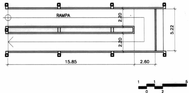
Fig. 2 – Planta rampa 2 – Escola A Fonte: Autor, 1998
