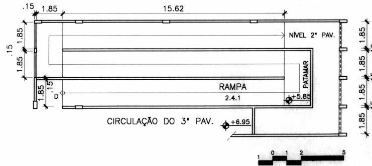
Fig. 5 – Planta rampa 2 – Escola C Fonte: Autor, 1998
