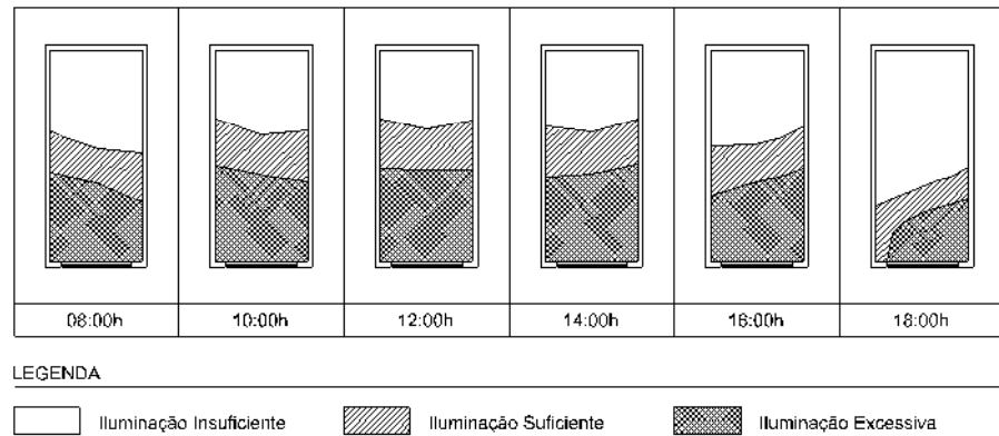
Fig. 1 Gráficos com curvas isolux para o Modelo A1 (2.80mx6.43m), sob condição de céu intermediário, no solstício de verão.
